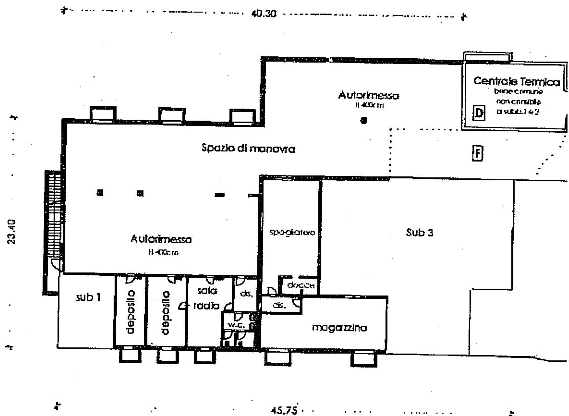
PIANTA PIANO PRIMO SOTTOSTRADA
