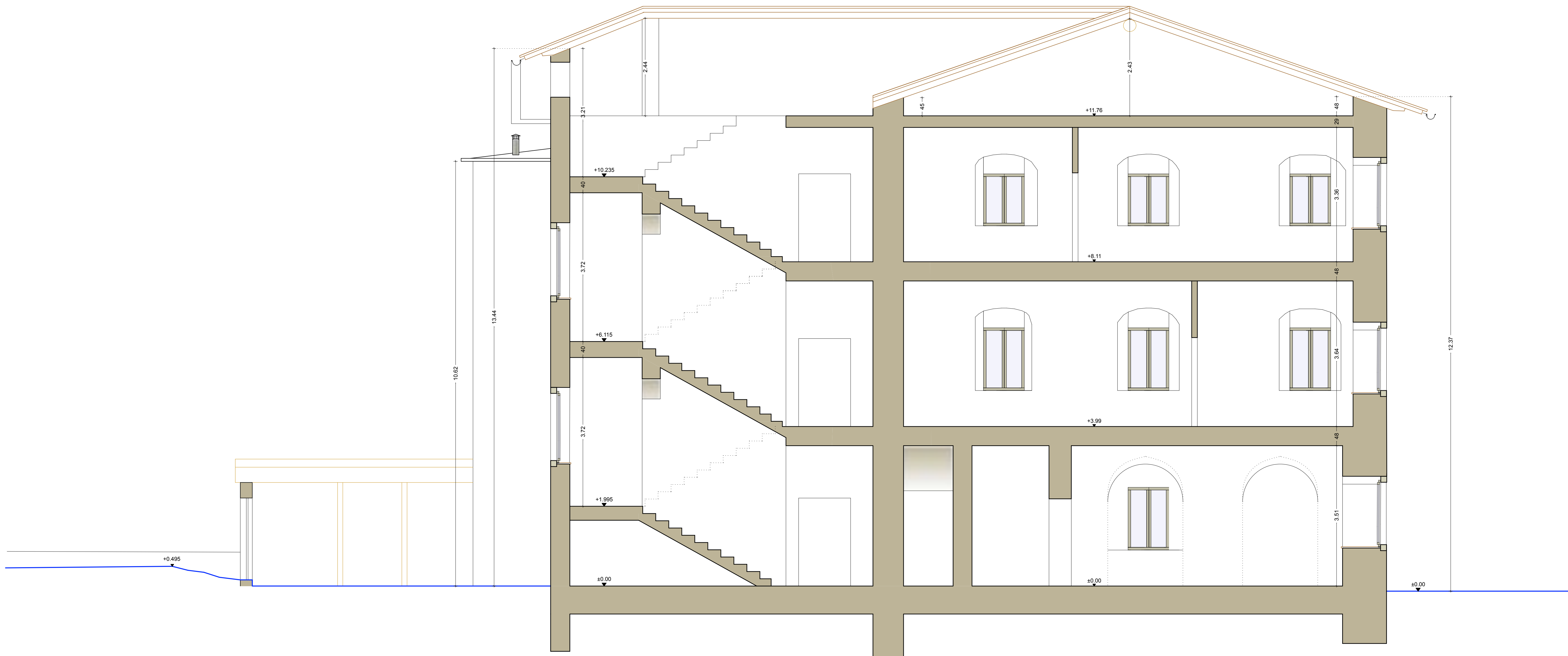
SEZIONE A - SCALA 1:50
