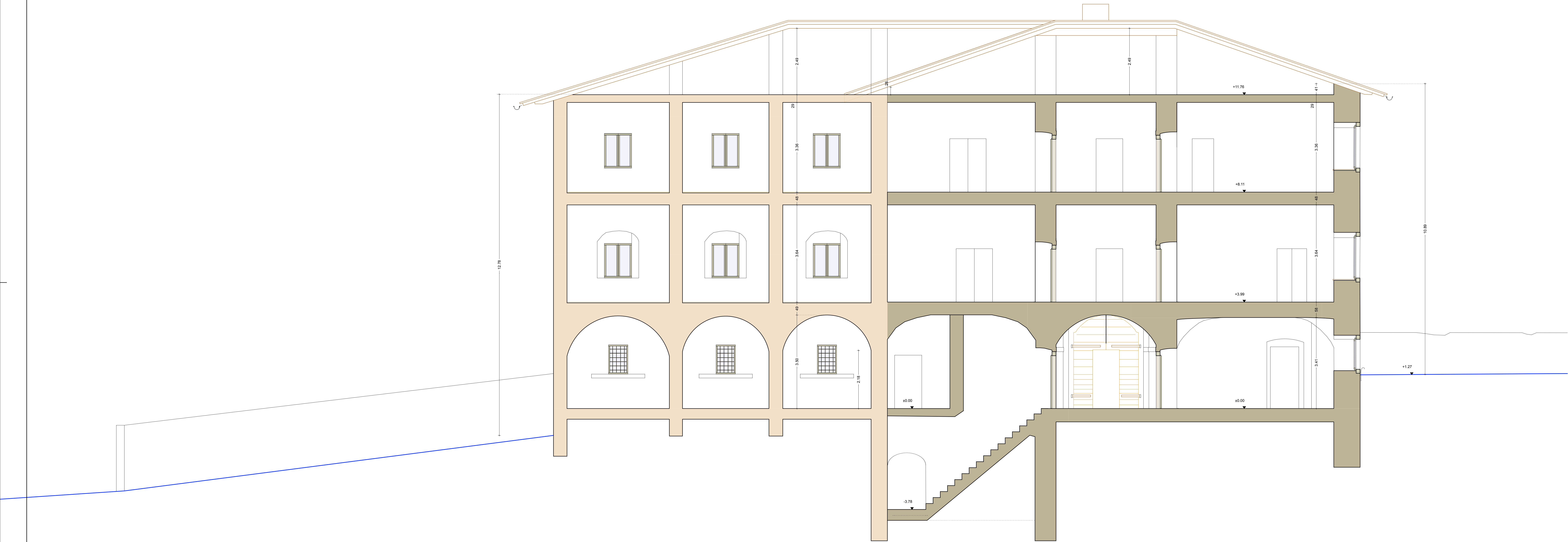
SEZIONE B - SCALA 1:50
